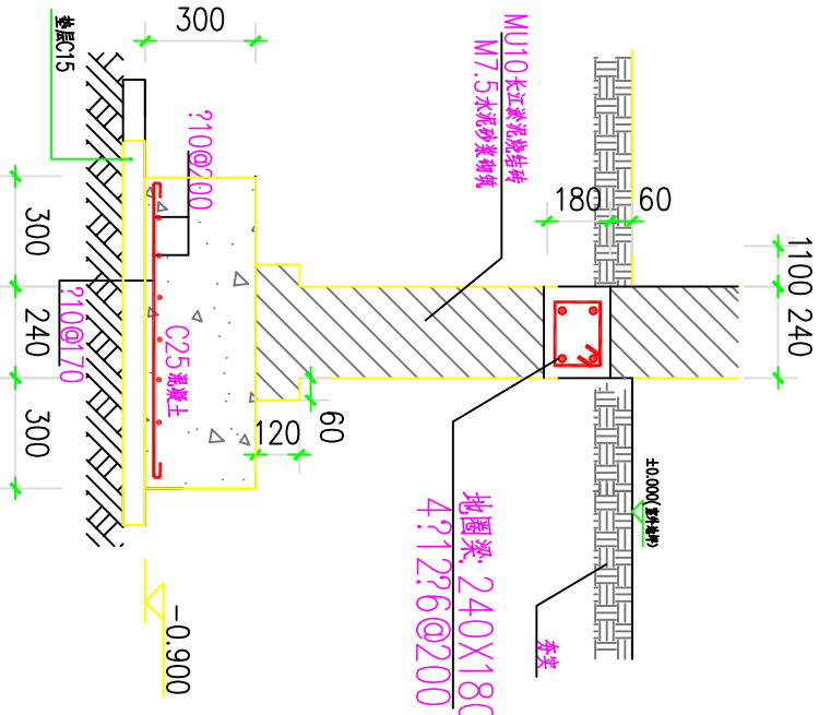
A-A剖面图 1:20
