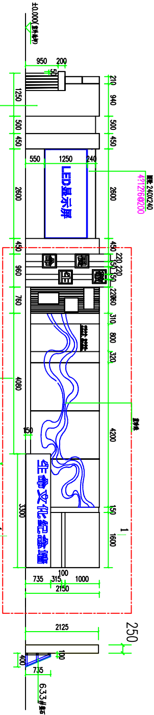
1-1剖面图 1:100
